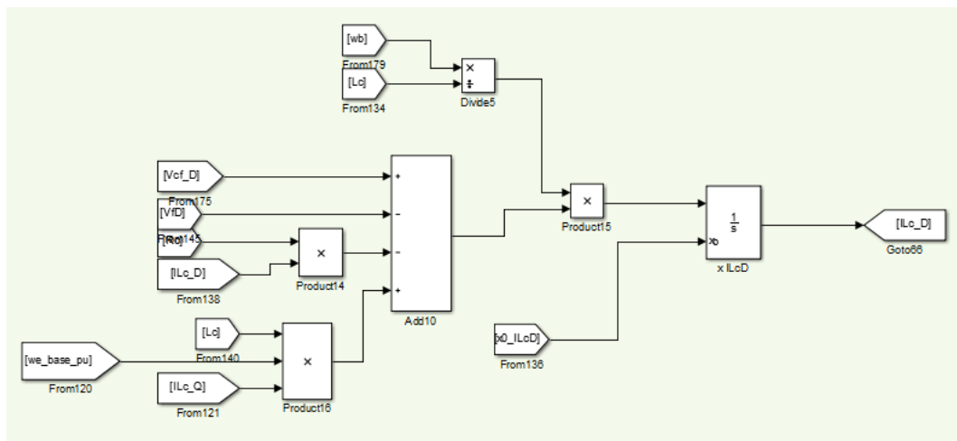
Figura A.27: Modelo dinámico del filtro LCL del modelo del inversor GFM Parte 4.
