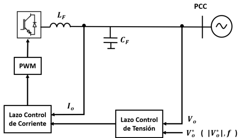
Figura 14: Modelo Control GFM.
