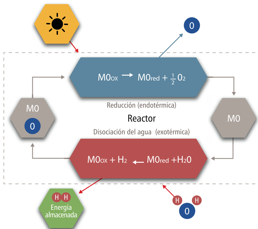
Figura 44: Esquema de un ciclo redox solar en dos pasos para la disociación del agua [153].
