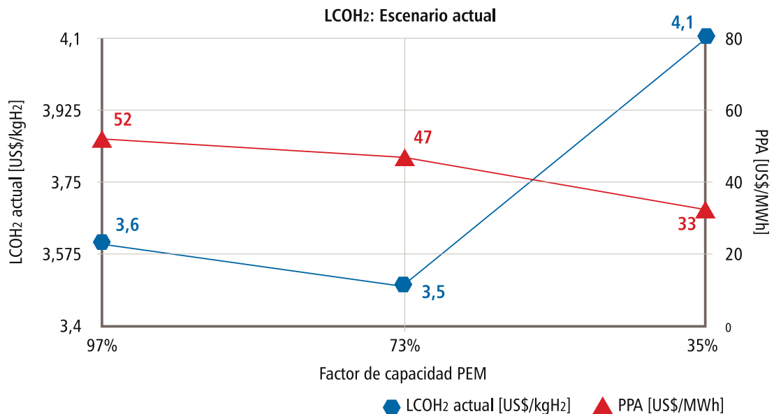
Figura 35: Costo nivelado de hidrógeno versus factor de capacidad del electrolizador PEM.
