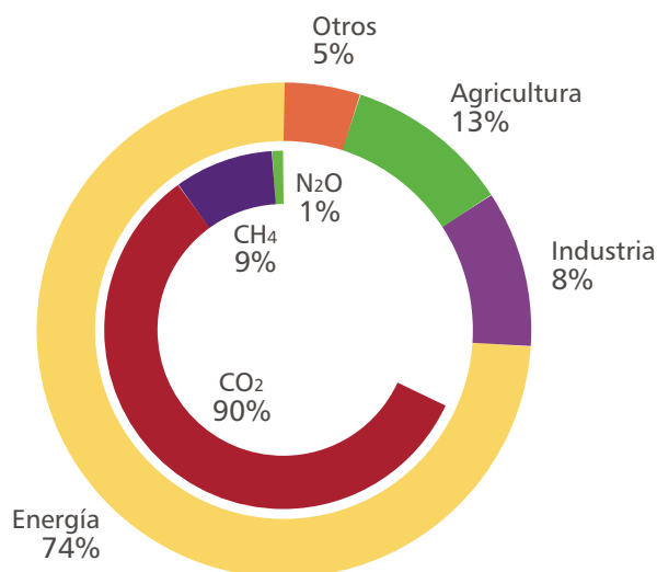
Figura 1: Porcentajes estimados de GEI antropogénico global, International Energy Agency (IEA).
