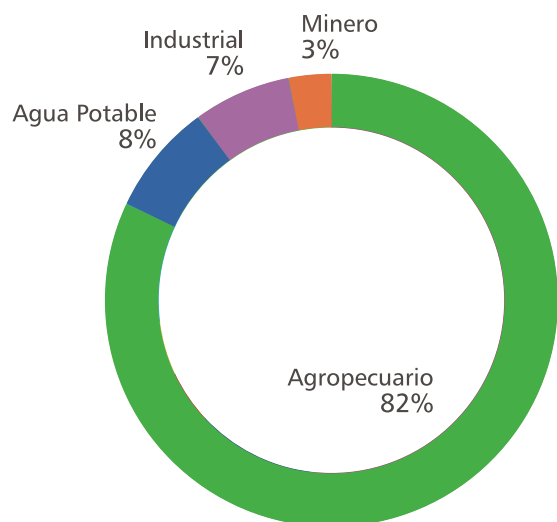
Figura 38: Consumos de agua en Chile por sector (2016) [147].
